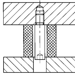
Mit Elastomer-Feder
